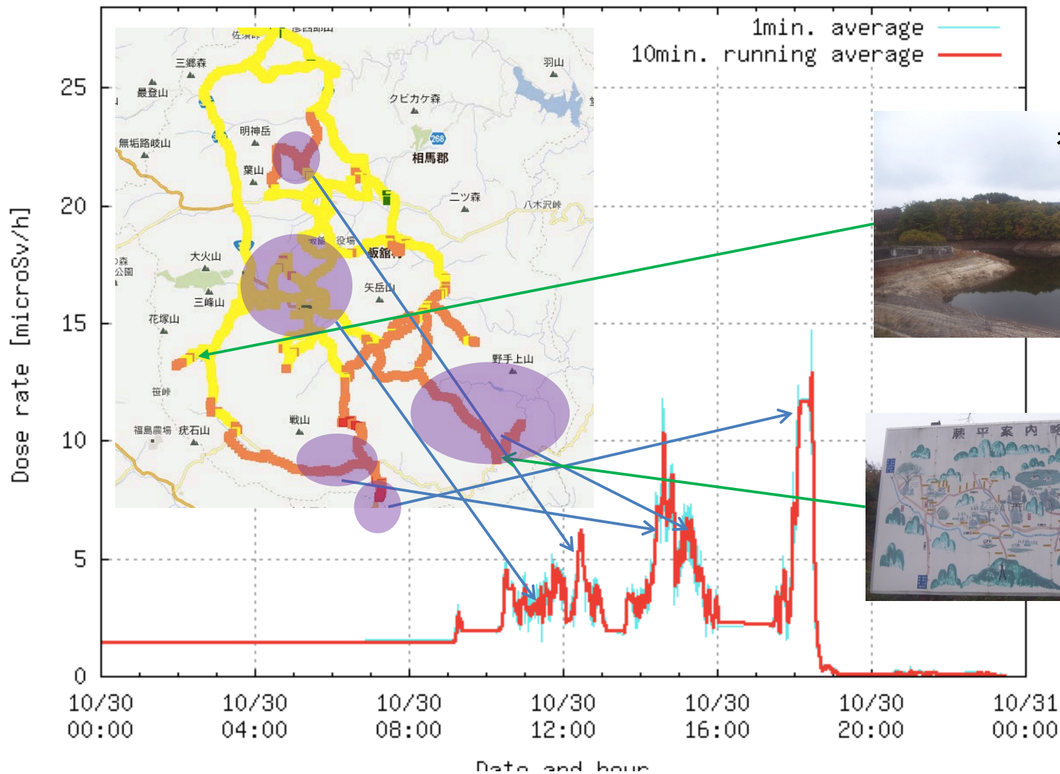
移動モニターの線量率の時間変化
