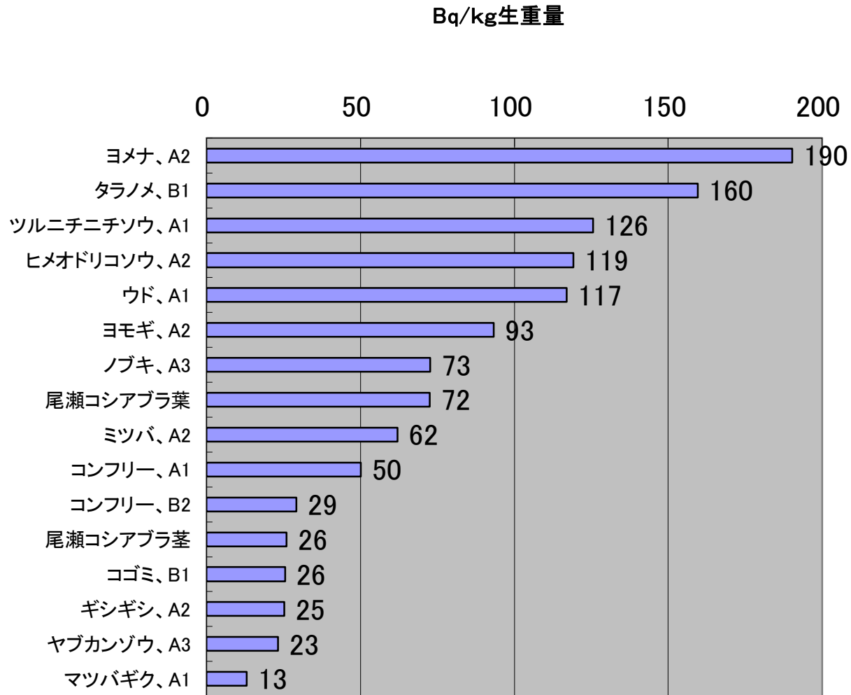
図1 飯舘村野草の放射性Cs濃度(2013/5/18-6/11採取)
